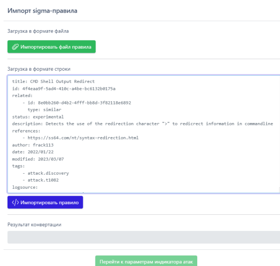
Рисунок 62 – Импорт Sigma-правила с помощью загрузки в формате строки для создания индикатора атаки
