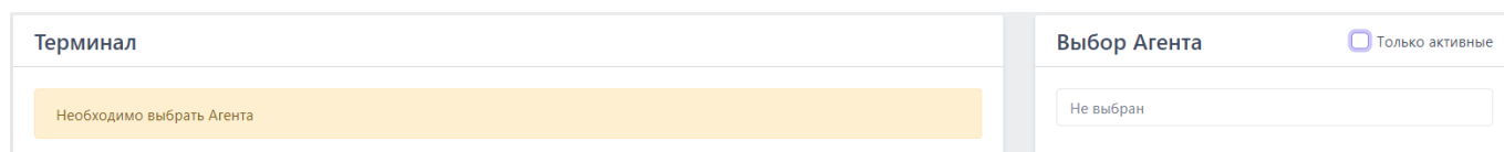
Рисунок 117 – Страница «Терминал»
