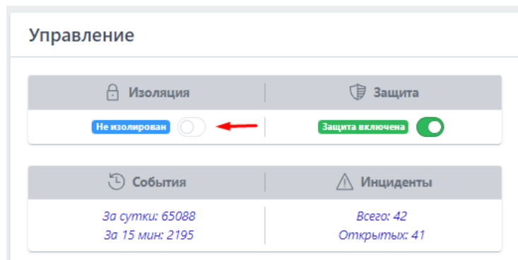
Рисунок 110 – Изоляция агента
