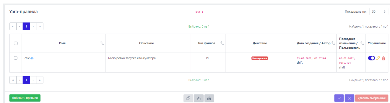
Рисунок 73 – Yara-правила
