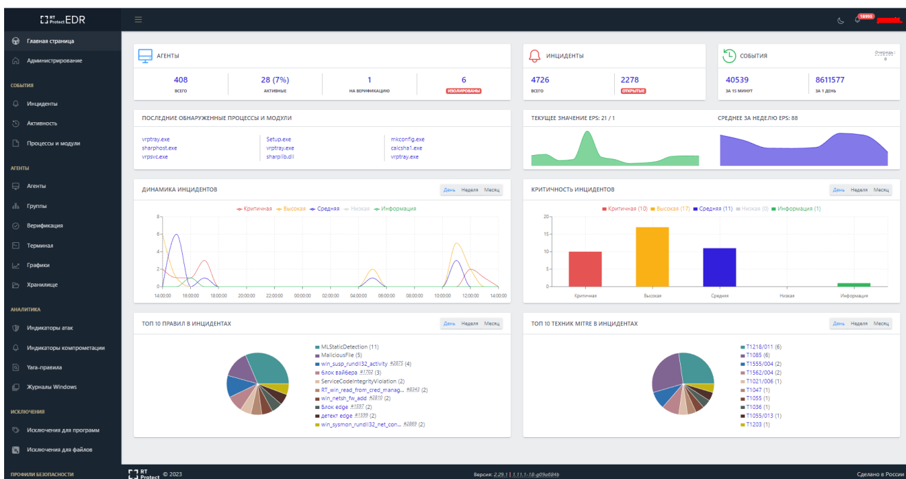
Рисунок 6 – Главная страница
