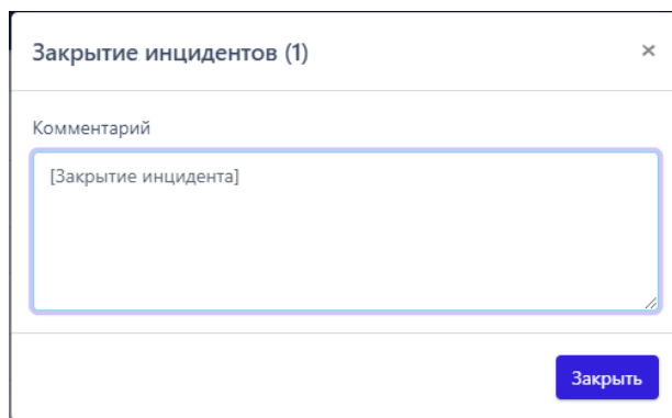
Рисунок 37 – Закрытие инцидентов
