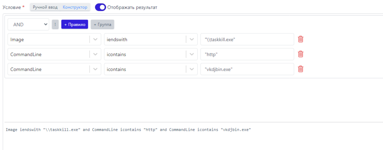
Рисунок 60 – Пример условия, написанного с помощью конструктора
