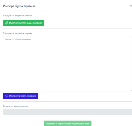
Рисунок 61 – Окно добавления индикатора с помощью импорта из sigma-правила
