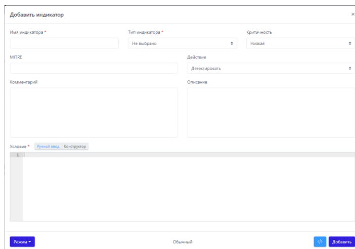
Рисунок 52 – Добавление индикатора
