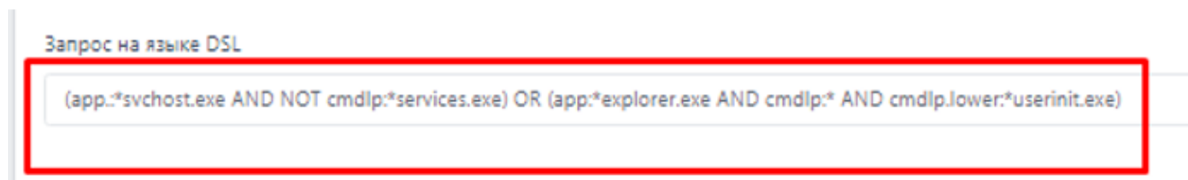
Рисунок 124 – Сложный DSL-запрос
