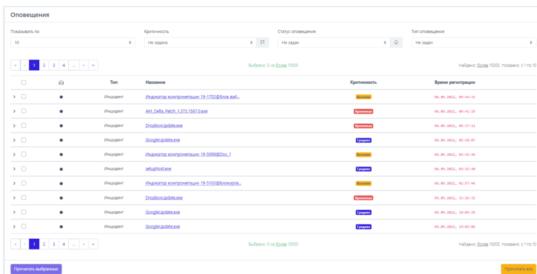
Рисунок 12 – Окно «Оповещения»
