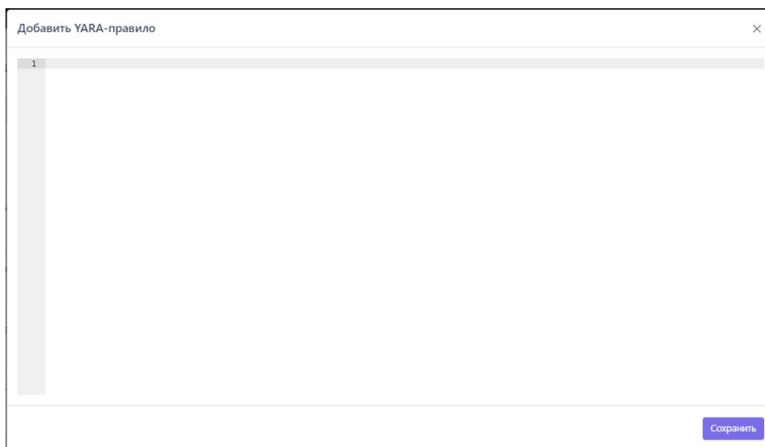
Рисунок 74 – Добавление Yara-правила
