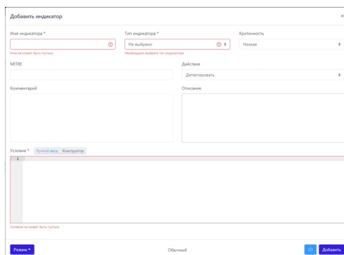
Рисунок 53 – Вид окна при добавлении индикатора с незаполненными полями
