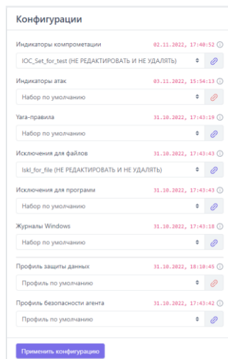
Рисунок 112 – Настройка конфигурации для агента
